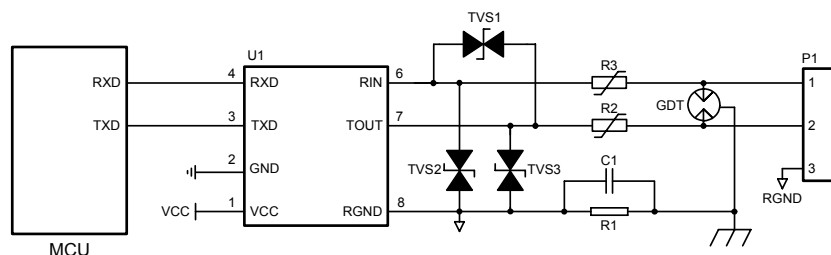
图 2 推荐应用电路图
