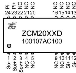
图 4.2 引脚分布图
